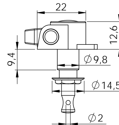
Untersicht bottom view
