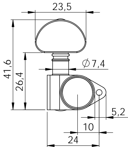
Seitenansicht von links side view left
