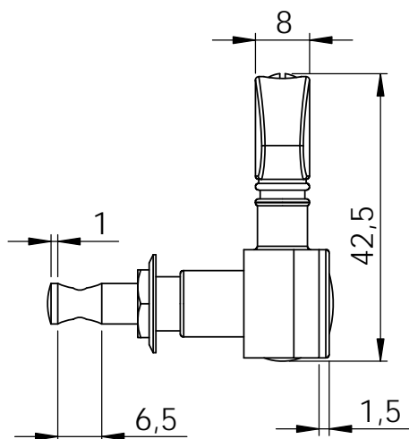
Seitenansicht von links side view left
