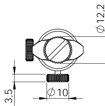
Seitenansicht von links side view left
