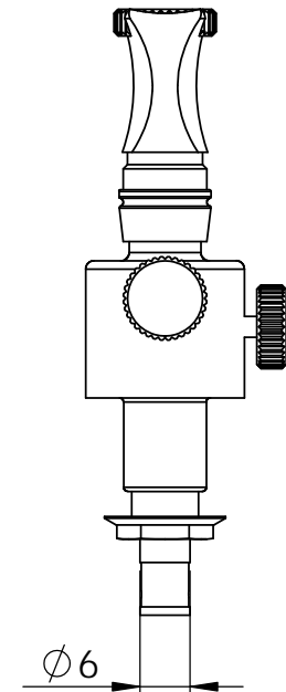
Seitenansicht von rechts side view right
